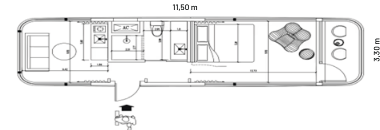
Wohnfläche LIU ca. 38 m 2
